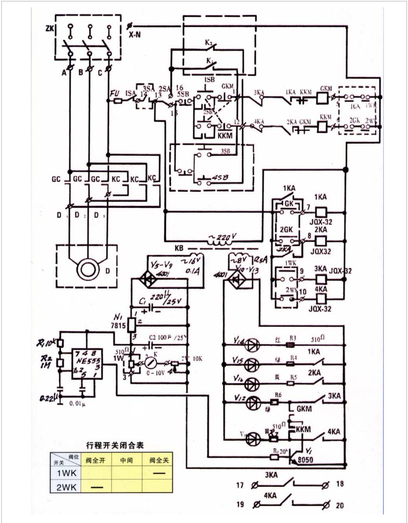
DFK-5/DFK-6/DFK-7/DFK-8 型电动阀门控制器 电气原理图
